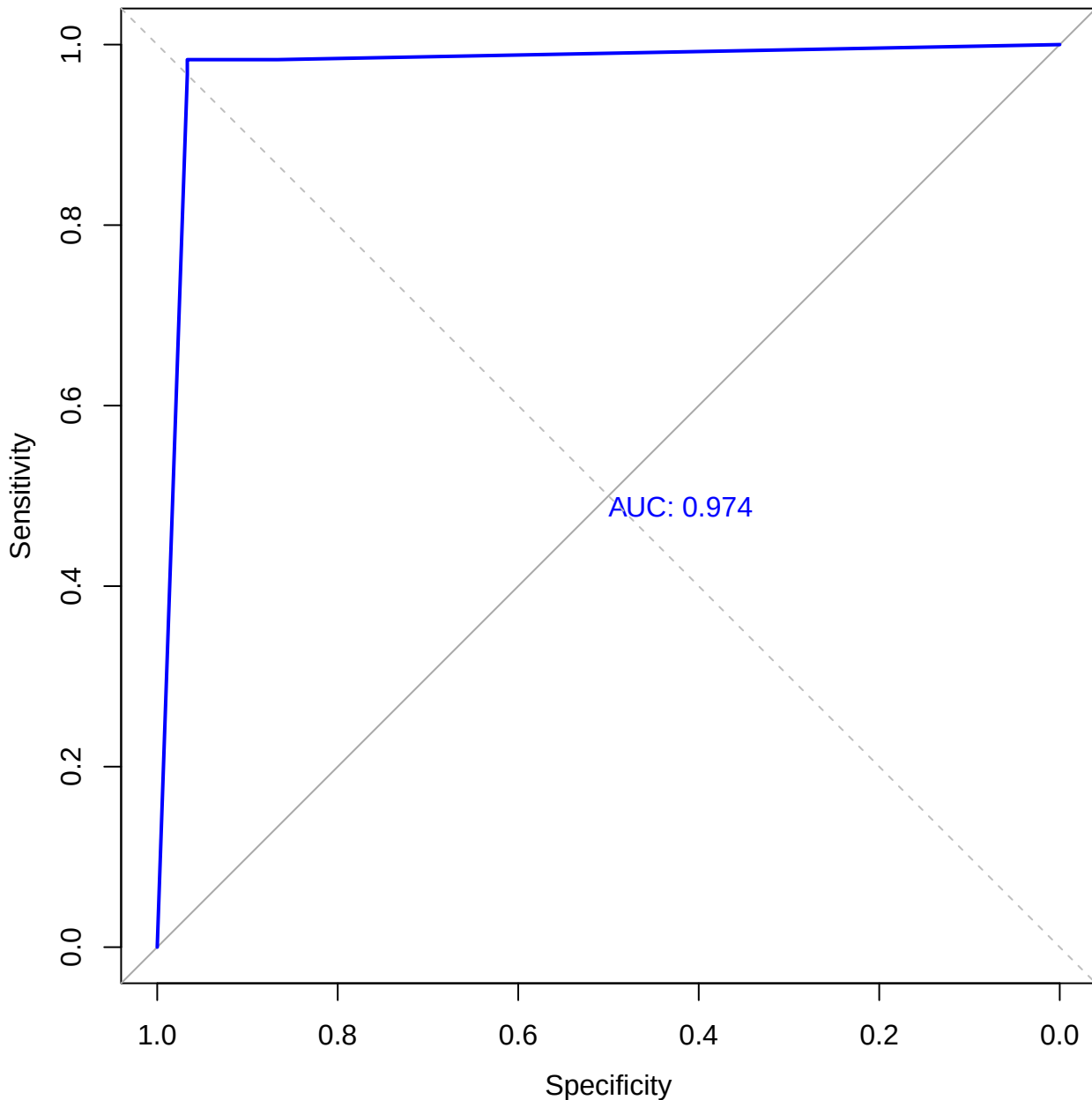
Curva ROC – Clasificación Binaria (Bueno vs No Bueno)
