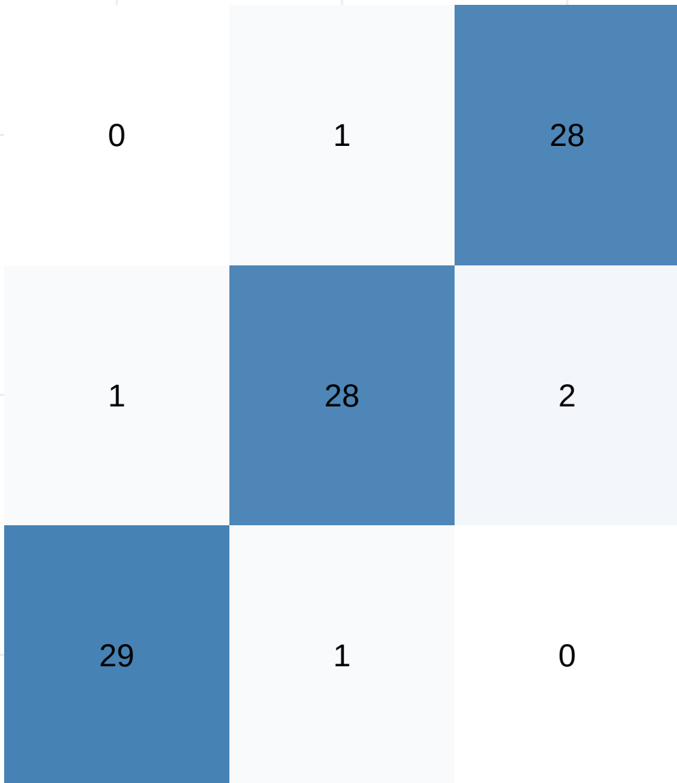
Matriz de Confusión – Regresión Logística Multinomial
